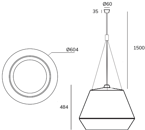
TE SUD Ø600
