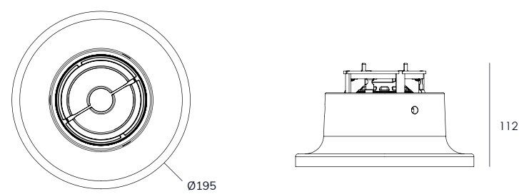
EN G53 Ø195
