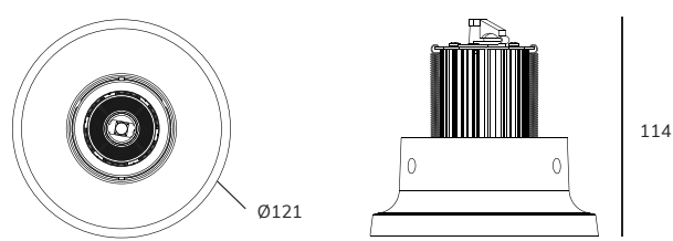
EN EL51 Ø121
