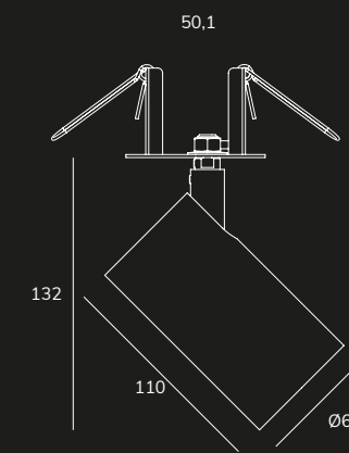
WHEEL TE SM GZ10 Ø60
